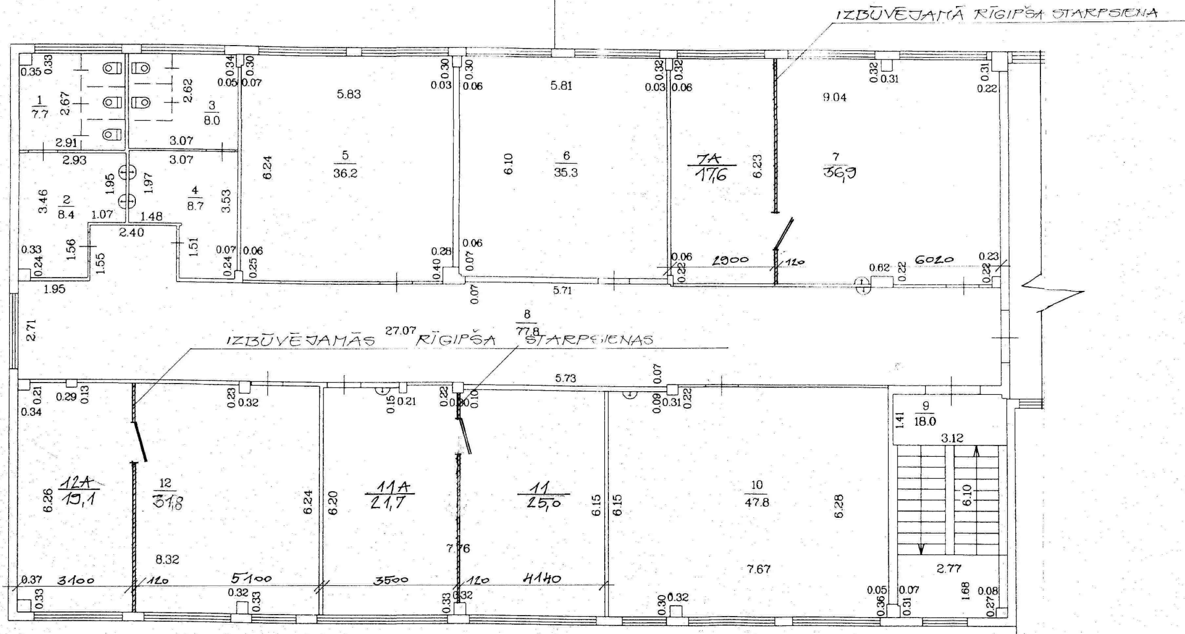
2. STĀVA PLĀNA FRAGMENTS M 1:100
